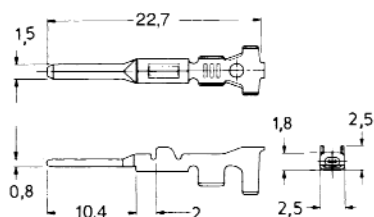
Contatto maschio Tab Contact
