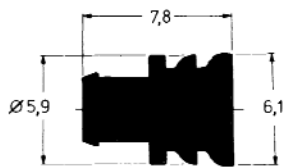
Tappo per cavità Cavity plug
