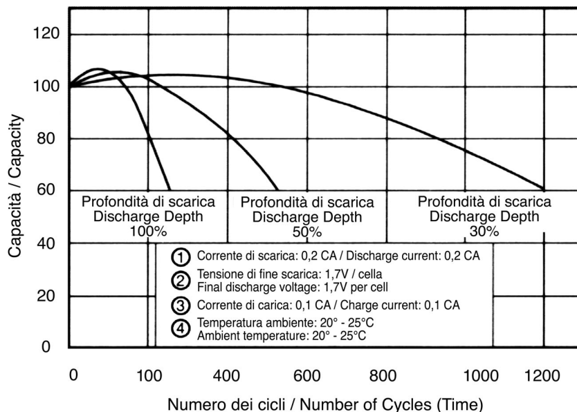
Numero di cicli in funzione della profondità di scarica
