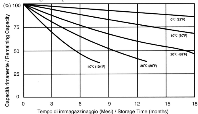
Autoscarica delle batterie in funzione della temperatura media di immagazzinaggio
