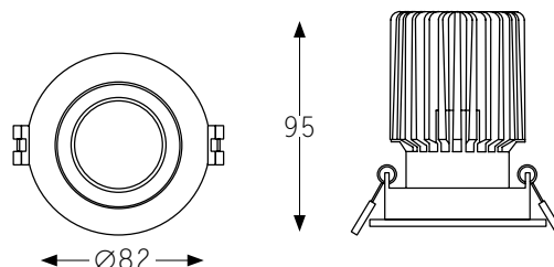
Disegno Tecnico
