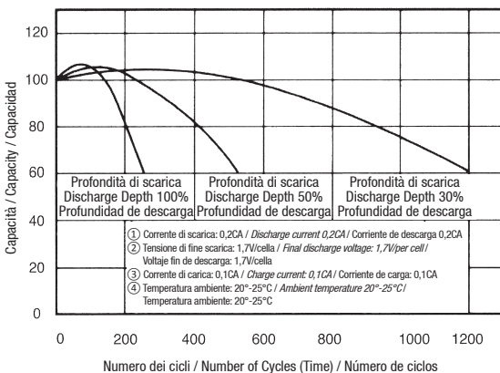
FIG.5 Numero di cicli in funzione della profondità di scarica. Relationship between cycle service life and the depth of discharge. Número de ciclos en función de la profundidad de la descarga.
