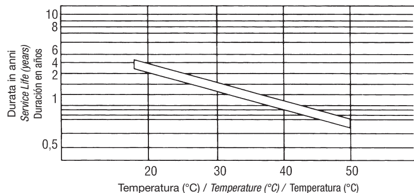
FIG.6A Vita in tampone delle batterie da 0,8Ah to 18 Ah. Float service life of battery from 0,8Ah to 18Ah. Vida en modo respaldo de las baterías desde 0,8Ah hasta 18 Ah.
