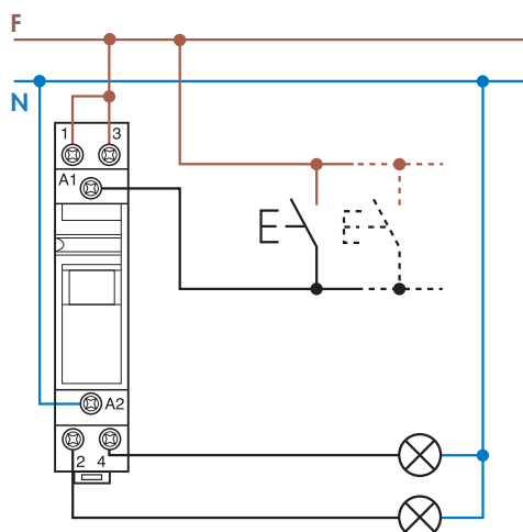
Esempio: tensione di alimentazione 230 V AC.
